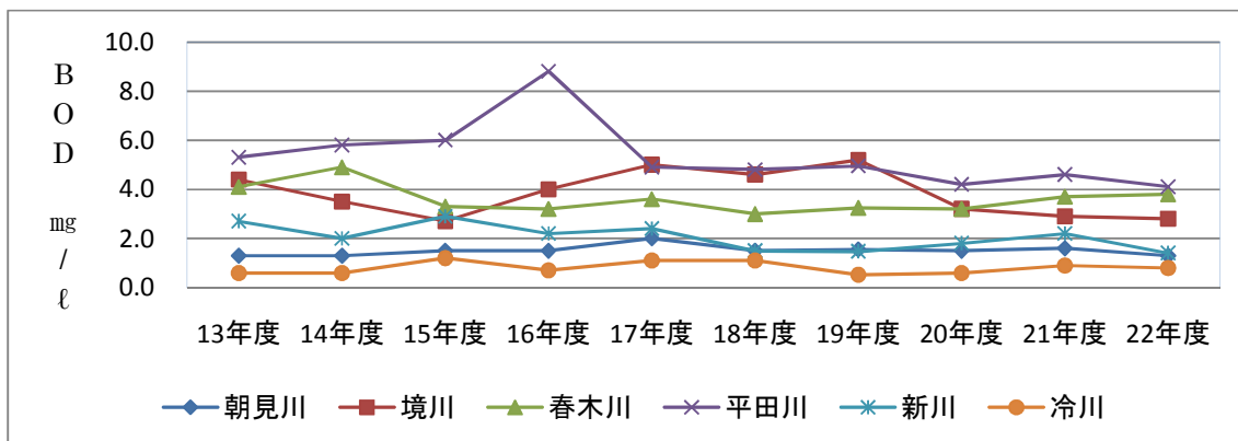
図表 2.15 市内主要6河川のBOD濃度の各年度の経年変化
