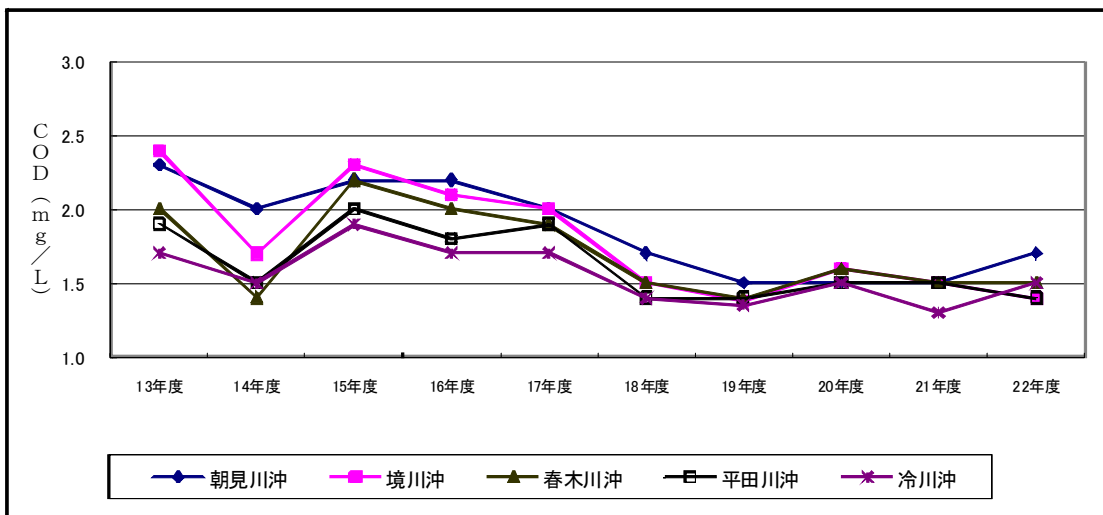
図表 2.16 別府湾地先海域 5 定点の COD 濃度の各年度の経年変化
